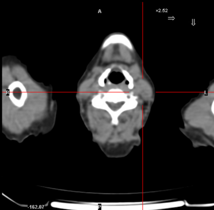
CT Transaxials
