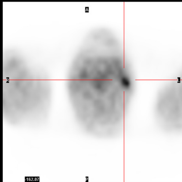
PET Transaxials
