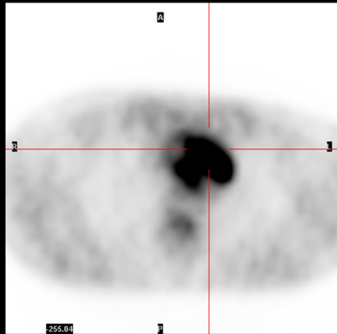
PET Transaxials
